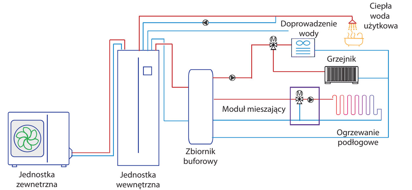
Układ 1: Układ z systemem All-In-One, wykorzystujący moduł mieszający
