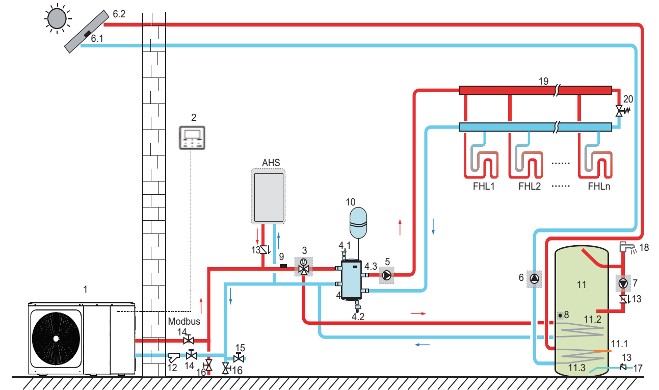
Układ 3: Układ z systemem monoblok, wykorzystujący funkcję sterowania kolektorami słonecznymi
