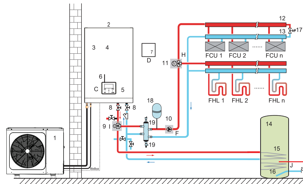
Układ 2: Układ z systemem split, wykorzystujący klimakonwektory dla chłodzenia pomieszczeń
